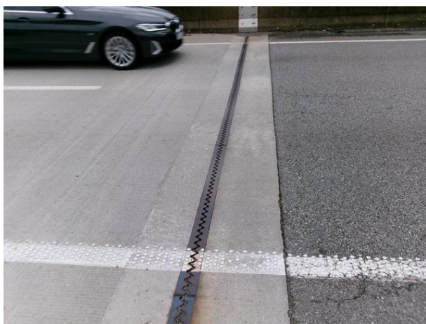
신축이음
